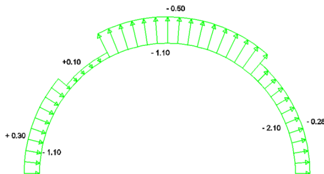
Figura 13. Corte esquemático. Perfil de presiones y succiones sobre cubierta
