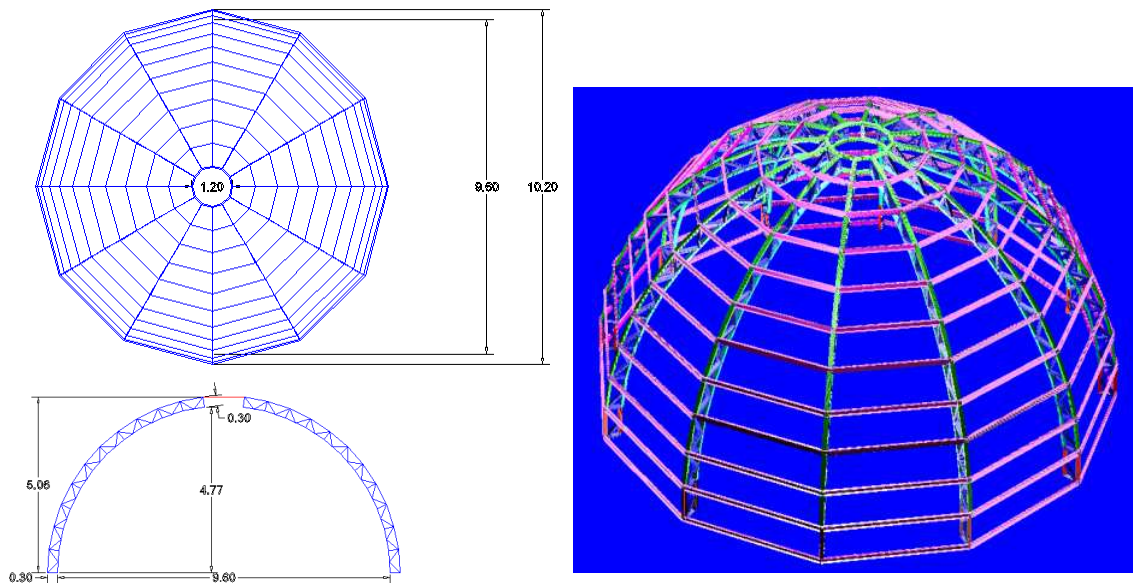
Figura 14. Planta, alzado y perspectiva del modelo de la cúpula para Strap
