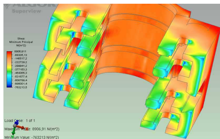
Figura 6. Tensiones de compresión en bases de muros
