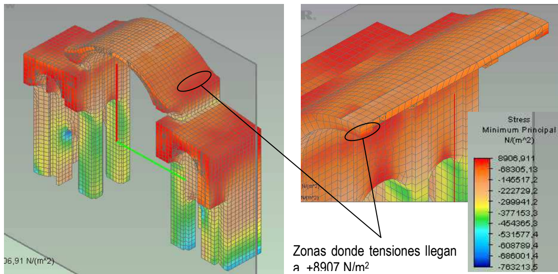
Figura 5. Tensiones de Compresión
