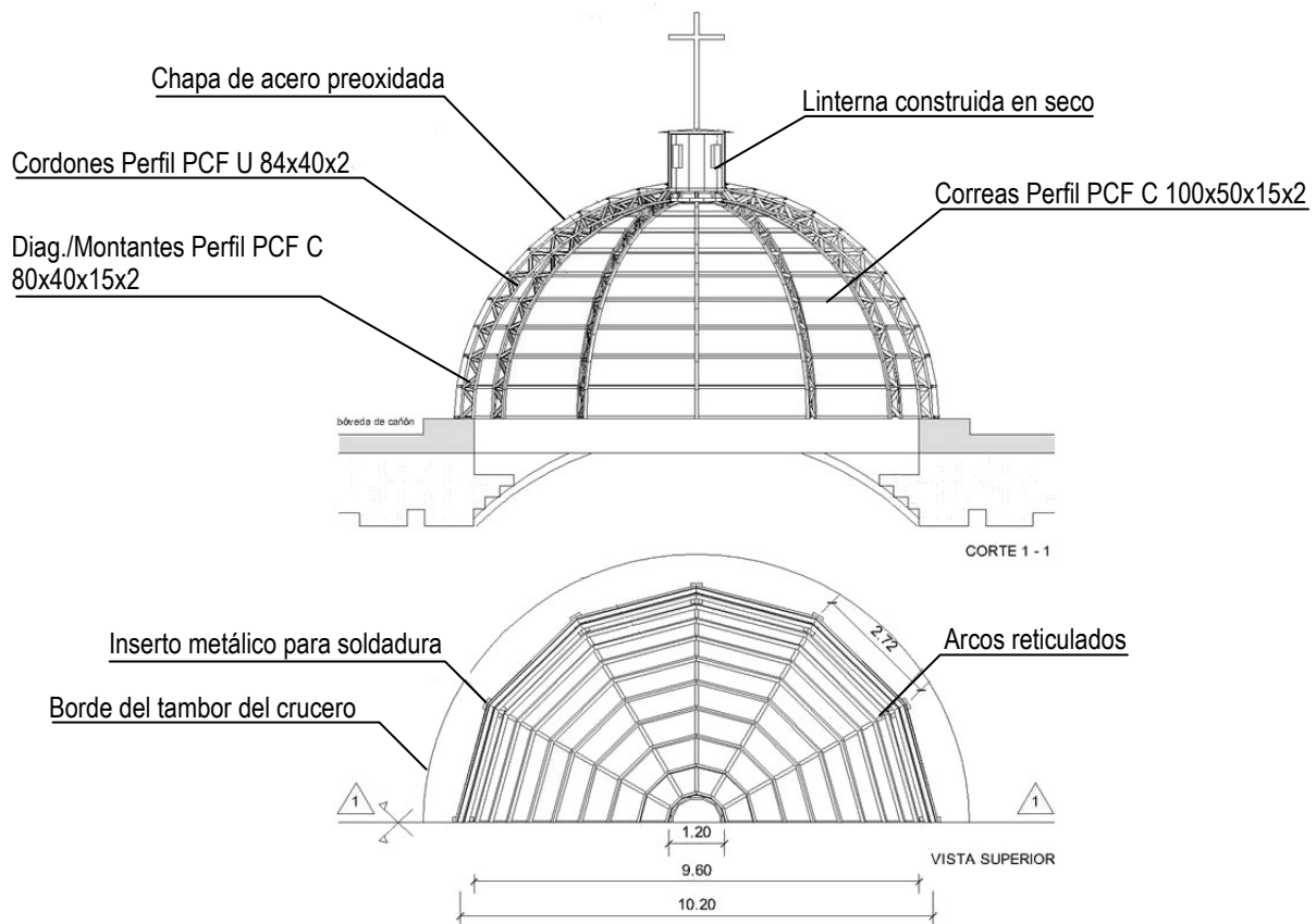
Figura 11. Planta y Corte de la cúpula proyectada
