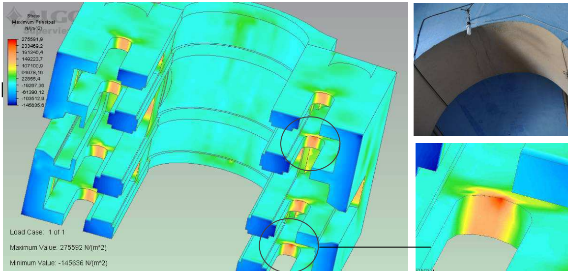
Figura 9. Zonas de tracciones en arcos dinteles
