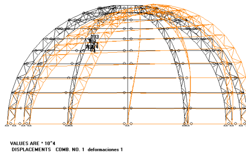
Figura 15. Deformaciones globales con cargas de viento
