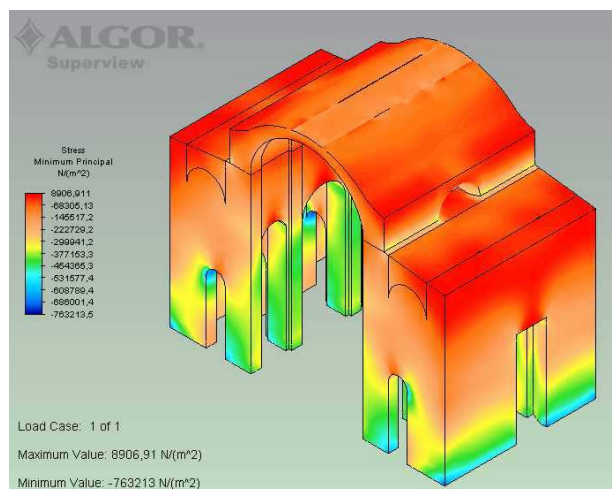
Figura 4. Tensiones de Compresión
