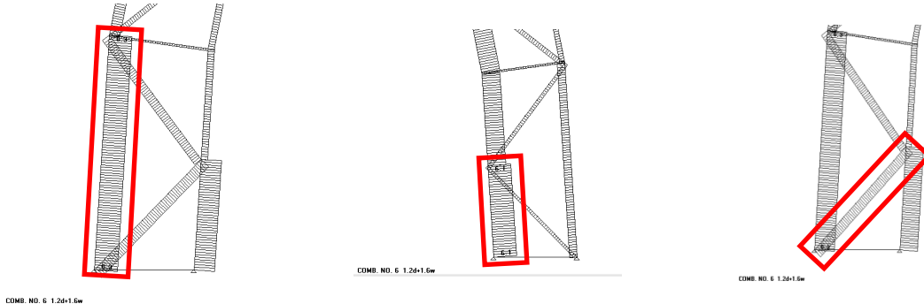
Figura 16. Barras con solicitaciones Normales máximas
