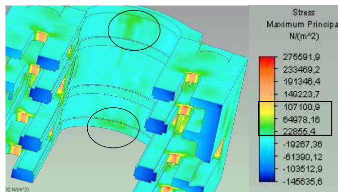
Figura 8. Zonas de tracciones en los nervios de la bóveda
