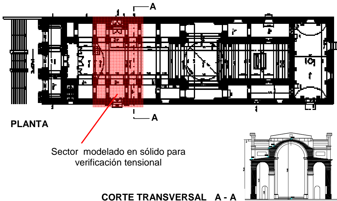
Figura 2. Planta y Corte transversal del Templo
