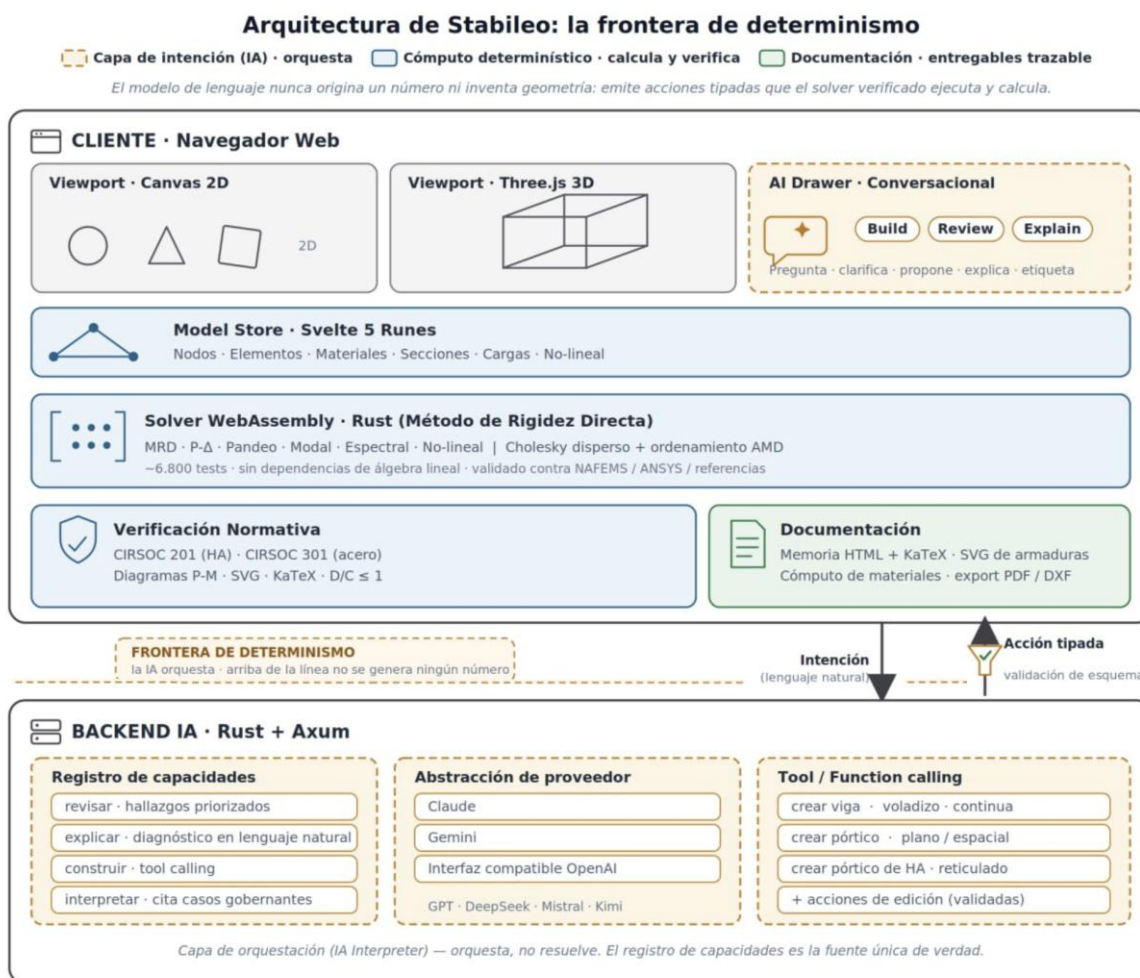
Figura 1. Arquitectura de Stableo: capas de intención (IA), cómputo determinístico y documentación, separadas por la frontera de determinismo.
